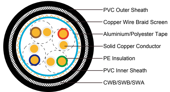
SF/UTP CAT5E
